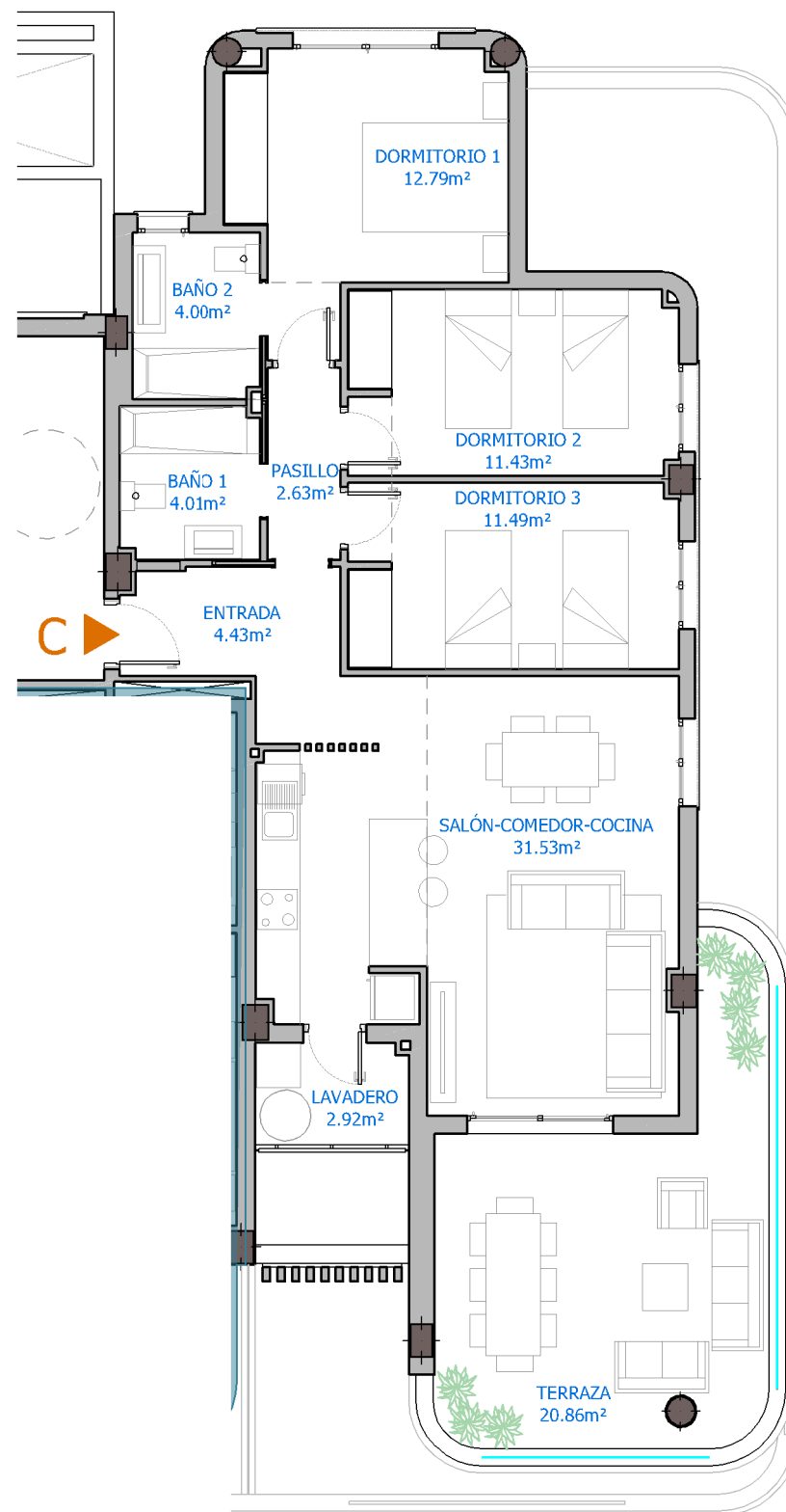
VIVIENDA C
