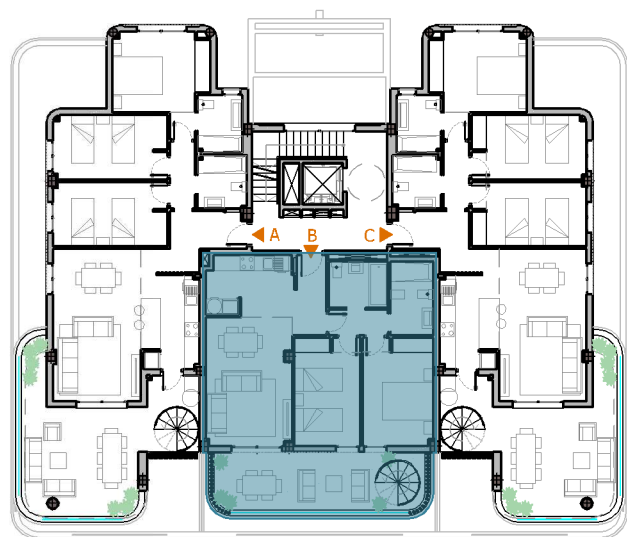
PLANTA TERCERA
