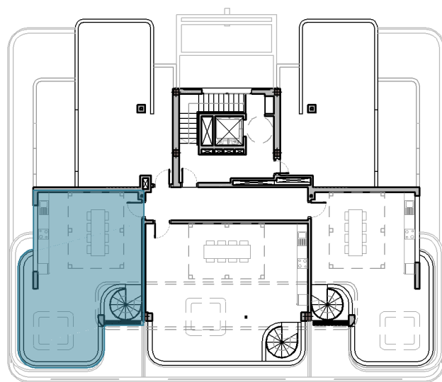
PLANTA SOLARIUM
