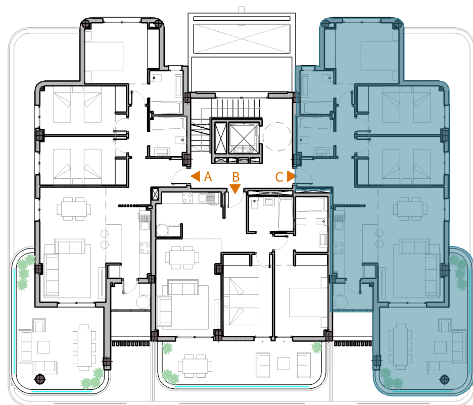
PLANTA PRIMERA
