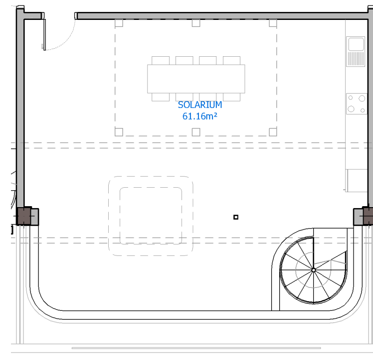
VIVIENDA B PLANTA SOLARIUM
